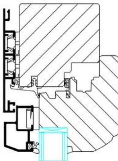
BFT HA IV 68 flächenbündig
